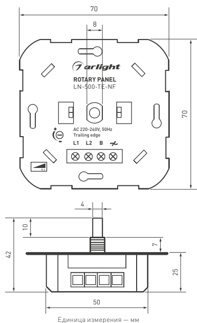
Единица измерения — мм Рисунок 1. Габаритные размеры панели LN-500-TE-NF.
